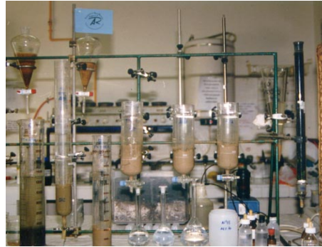
Foto 1: Reactores a escala laboratorio.
