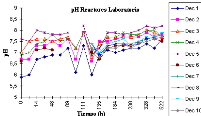
Figura 3: Evolución del pH en los reactores.
