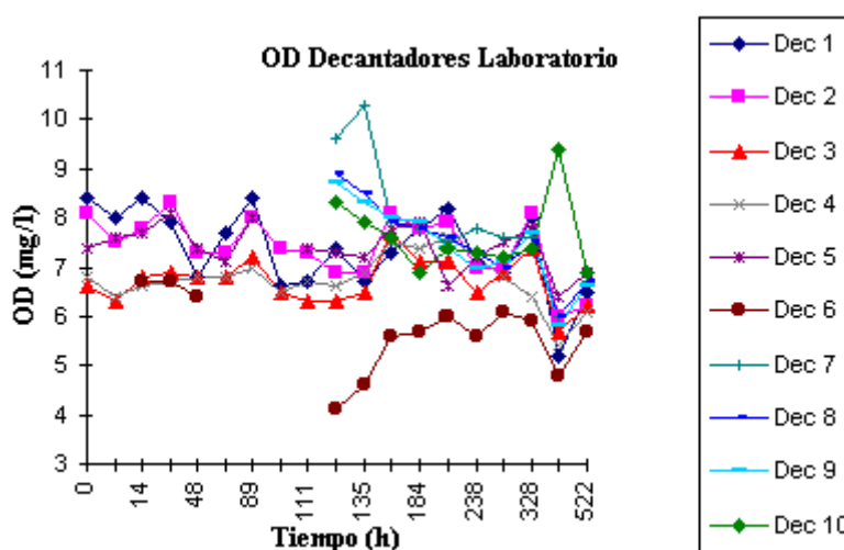
Figura 1: Evolución del oxígeno disuelto en los reactores.
