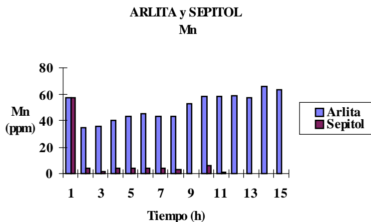
Figura 6.- Evolución en el contenido en Mn del agua con \text{pH}_i 7 al tratarla con arlita y sepiol.
