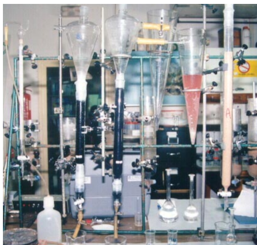
Foto 1: Ensayo en columnas de carbón activo y arcillas tratadas.
