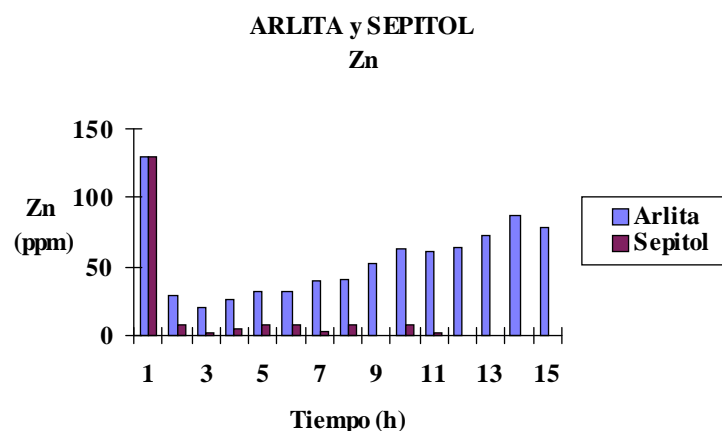
Figura 5.- Evolución en el contenido en Zn del agua con \text{pH}_i 7 al tratarla con arlita y sepiol.
