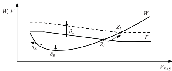
BILD 1: Abhängigkeiten von Schub F und Widerstand W von den Stellgrößen Schubhebel \delta_F , Bremsklappenhebel \delta_B und Klappenstellung \eta_K sowie der äquivalenten Fluggeschwindigkeit V_{EAS} ; Z_1 und Z_2 markieren getrimmte Zustände für zwei verschiedene Schubhebelstellungen
