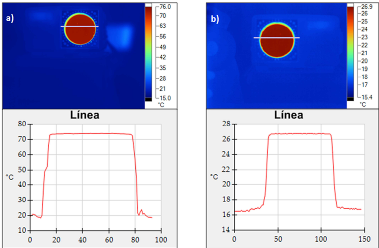
Figura 5. La imagen a) corresponde a la fuente, seteada en 75°C y la b) es la imagen del reflejo producido por una muestra espejada. Notar que las escalas de ambas imágenes son diferentes.
