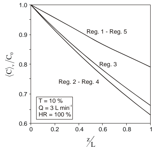
Figura 4. Concentración adimensional promedio, pesada en velocidades, para distintas alturas. Irradiación bilateral.
