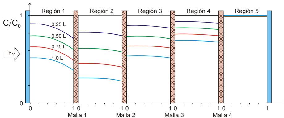
Figura 3. Perfiles de concentración adimensional. Irradiación unilateral. T = 10 \% ; Q = 3 \text{ L min}^{-1}
