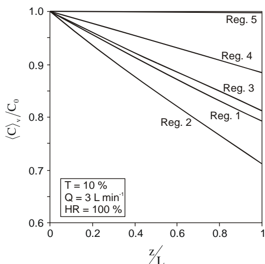
Figura 5. Concentración adimensional promedio, pesada en velocidades, para distintas alturas. Irradiación unilateral.
