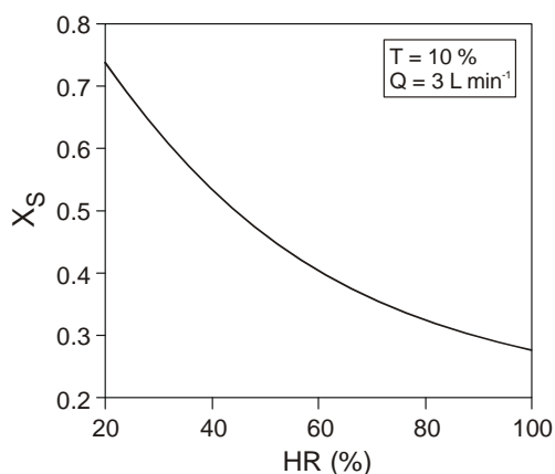
Figura 6. Conversión para humedades crecientes.
