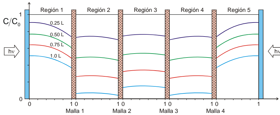
Figura 2. Perfiles de concentración adimensional. Irradiación bilateral. T = 10 \% ; Q = 3 \text{ L min}^{-1}
