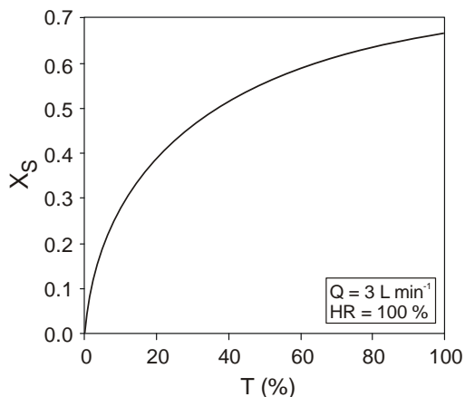
Figura 7. Conversión para irradiación creciente.
