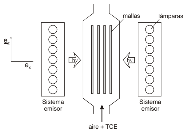
Figura 1. Reactor fotocatalítico y Sistema emisor.
