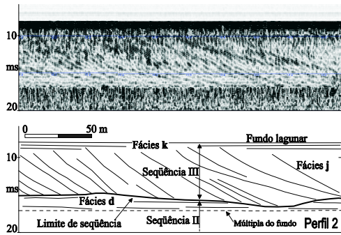
Figura 6 – Elementos arquiteturais identificados no setor nordeste do perfil 2 (ver na figura 1 a localização do registro sísmico): fácies d, j, e k; seqüências II e III. Profundidade em tempo de ida e volta, em milissegundos (ms).
