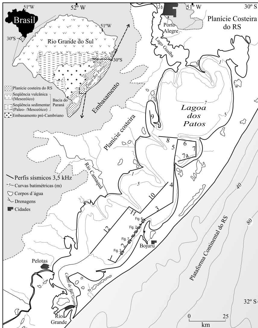
Figura 1 – Mapa de localização da área de estudo. Linhas de 1 a 12 são perfis sísmicos de 3,5 kHz levantados no interior da Lagoa dos Patos. No mapa é indicada a posição dos registros sísmicos das figuras 2, 3, 6 e 7, discutidas no texto.
