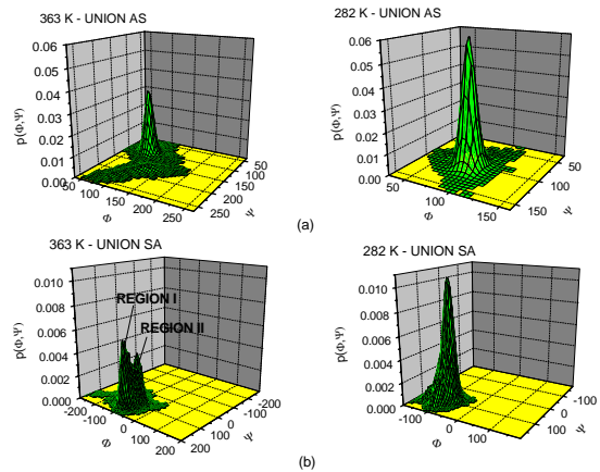
Figura 2: a) funciones de probabilidad p(\phi, \psi) para la unión AS a T=363K y 282K (arriba) y b) idem para la unión SA (abajo)
