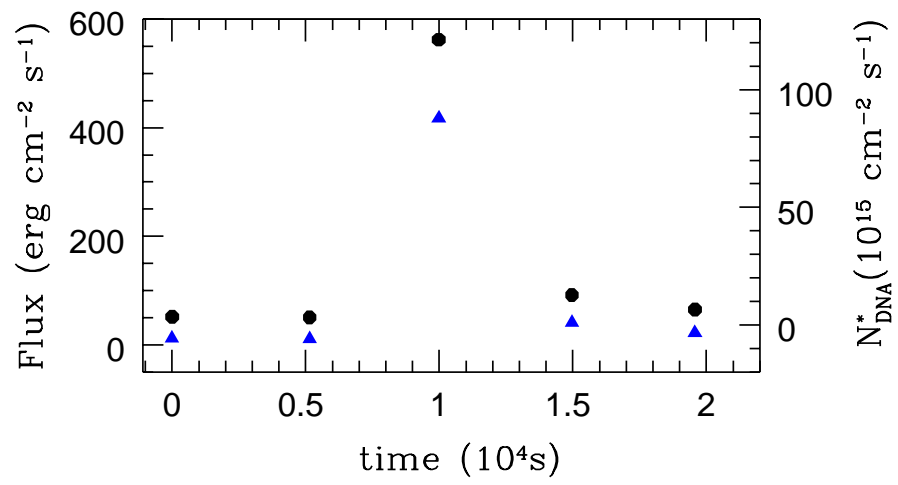
Fig. 3. Buccino et al. , 2007. Flare in AD Leo.
