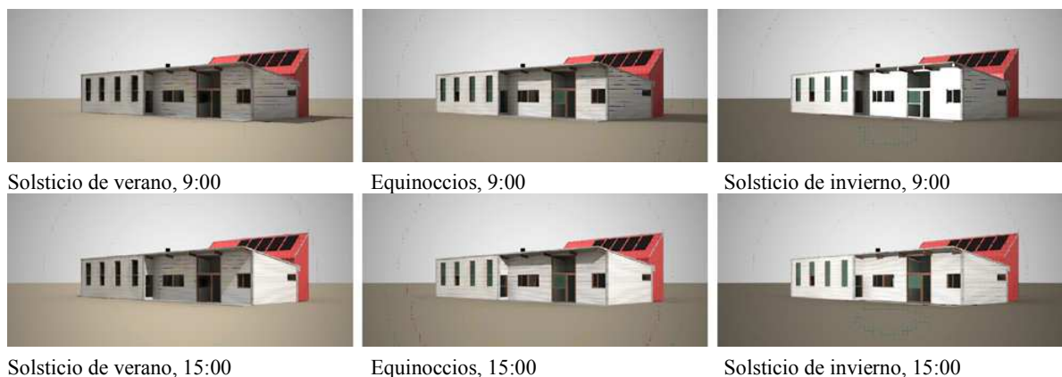
Figura 3: Estudios de asoleamiento en la fachada norte
