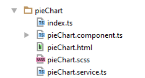
Figure 22 : Structure et fichiers d'un package contenant un Component
