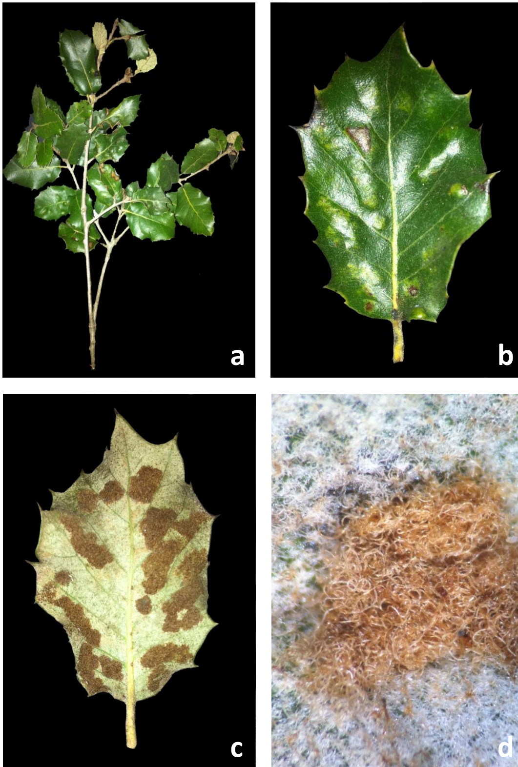
Figura 4. Daño (eriosis) realizado por Aceria ilicis y A. trichophila a Quercus ilex , a) Vista general del daño en las hojas, b) Abultamientos en el haz de la hoja, c) Erineos en el envés de la hoja, d) Detalle de los tricomas (erineos).
