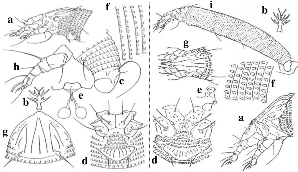
Figura 1. Principales detalles morfológicos de Aceria ilicis (izquierda, según Canestrini, 1890) y de A. trichophila (derecha, según Keifer, 1955). (a) gnatosoma en visión lateral, (b) detalle del empodio, (c) parte distal, con detalle de los lóbulos anales y las setas h1 y h2, (d) Platos coxales y región genital de la hembra, (e) Espermatecas, (f) Detalle de los micro tubérculos, (g) Detalle del escudo predorsal, (h) Patas II, (i) Eriófido en visión lateral.
