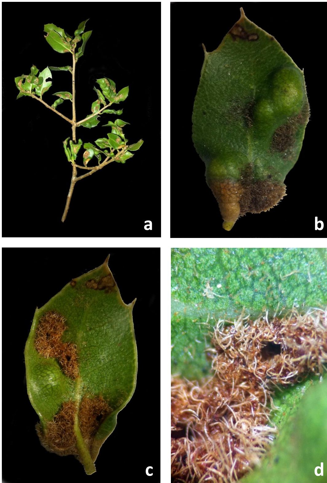
Figura 3. Daño (eriosis) realizado por Aceria ilicis a Quercus coccifera . a) Vista general del daño en las ramas, b y c) Abultamientos y erineos en el haz y envés de la hojas, d) Detalle del crecimiento anormal de los tricomas (erineos).
