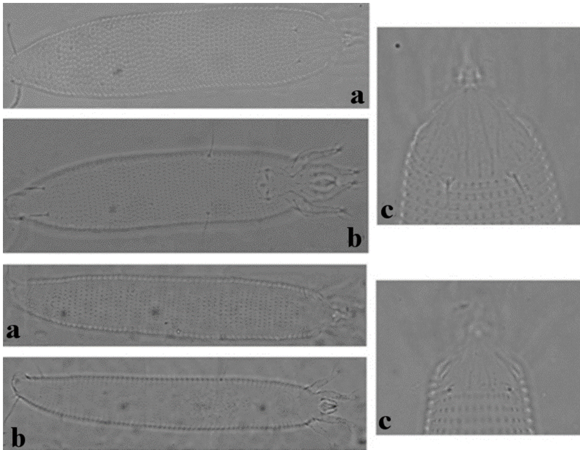
Figura 2. Vista dorsal (A), vista ventral (B) y detalle del escudo predorsal (C) de Aceria ilicis (sección superior) y A. trichophila (sección inferior).
