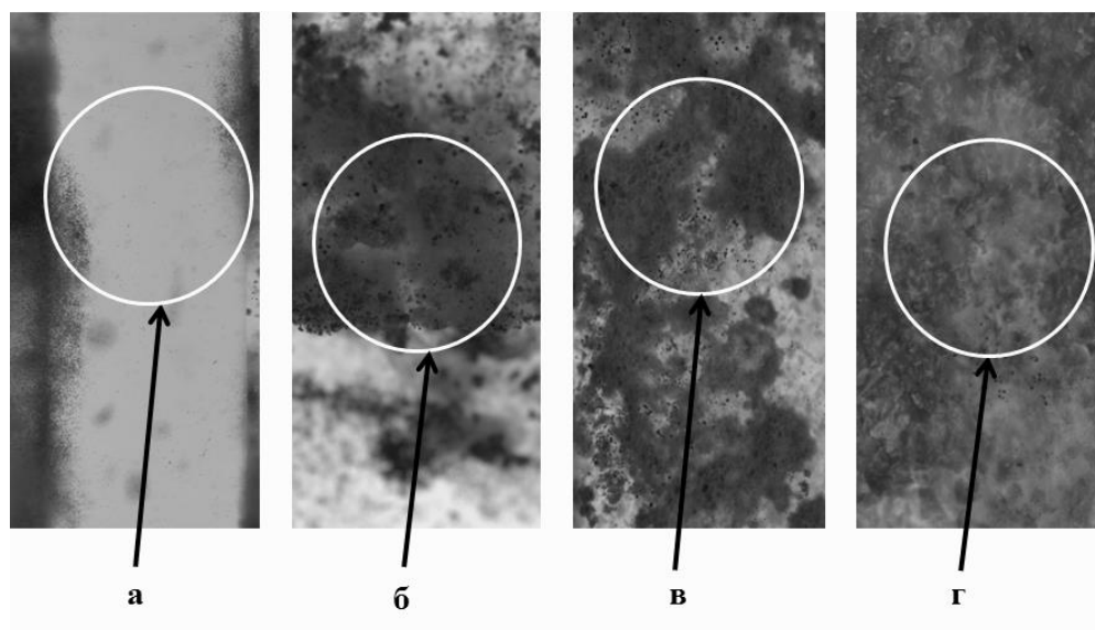
Рис. 4. Оптические фотографии ПЭ (а), композитов ПЭ/кератин при соотношении компонентов 90/10 (б), 60/40 (в) и кератина (г) после воздействия на них плесневых грибов
