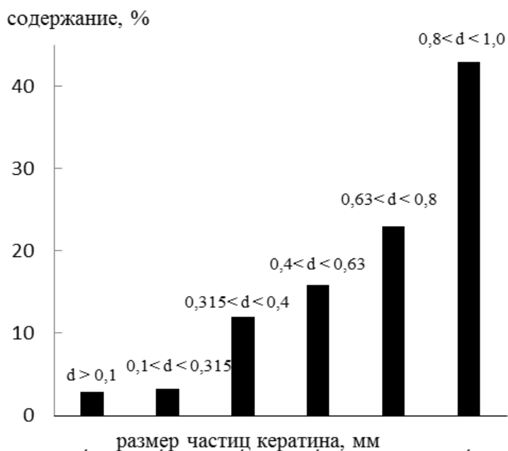
Рис. 1. Дисперсный состав кератина, полученный методом вибрационного рассева
