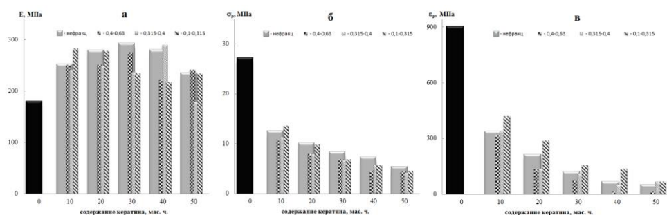
Рис. 3. Зависимость модуля упругости (а), предела прочности (б) и удлинения при разрыве (в) от содержания кератина в композите и его дисперсности
