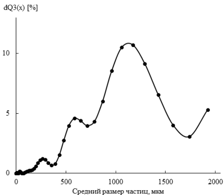
Рис. 2. Дисперсный состав кератина, полученный методом лазерной дифракции
