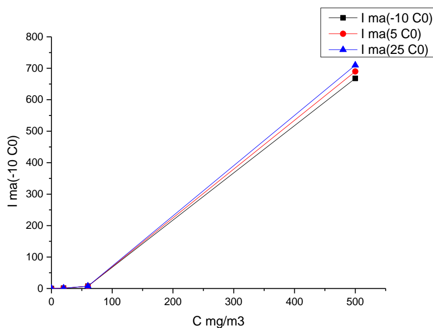
Рис. 4. Общий схематичный график зависимости силы тока от концентрации аммиака и температуры.
