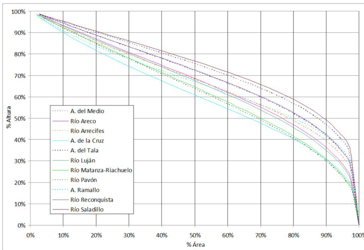
Figura2. Curvas hipsométricas determinadas para los ríos y arroyos seleccionados.
