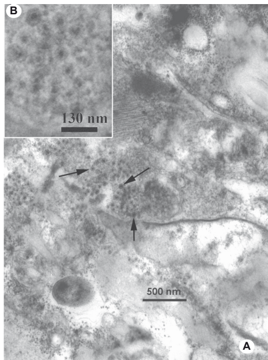
FIG. 1 - A. Micrografía electrónica de un corte ultrafino de glándula salival de Tagosodes orizicolus alimentado sobre trigo enfermo con Mal de Río Cuarto virus . Las flechas indican la presencia de partículas virales típicas de la Familia Reoviridae . Magnificación 10.000x; B. Detalle de A.
