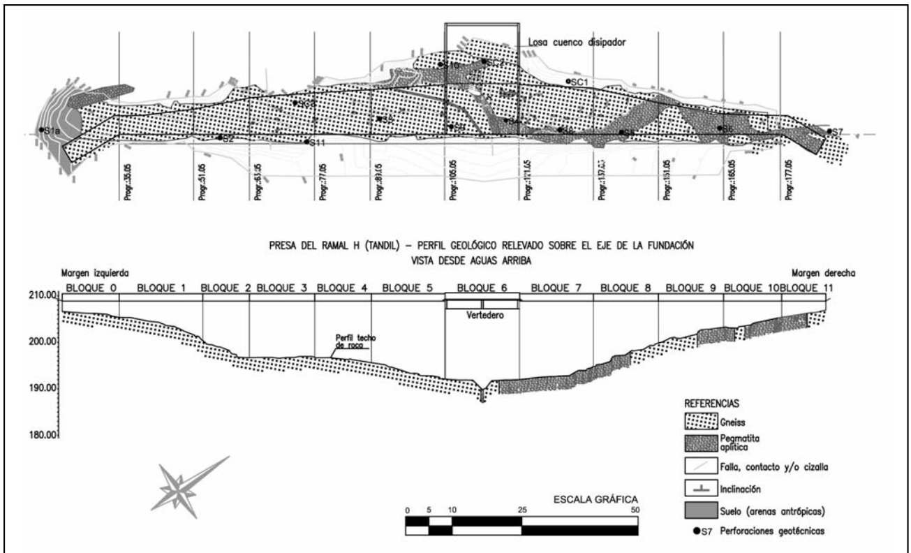
Figura 1. Ramal H. Plano Relevamiento y Perfil Geológico.
