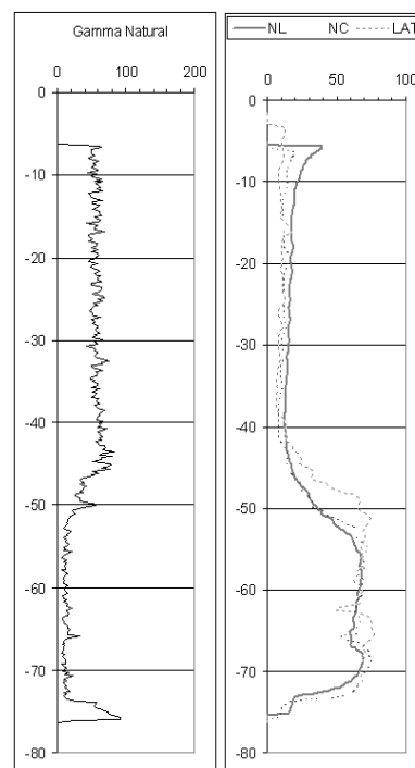
Figura 2. Perfilaje geofísico.
