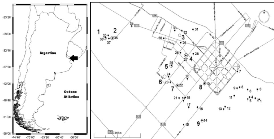
Figura 1. Ubicación del área de estudio, de los pozos con perfilajes geofísicos y SEV.
