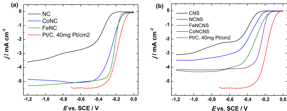
Joonis 6. Hapniku redutseerumise polarisatsioonikõverad erinevate materjalidega modifitseeritud klaassüsinikelektroodidel hapnikuga küllastatud 0,1 M KOH lahuses. v = 10 \text{ mV s}^{-1} , \omega = 1900 \text{ min}^{-1} . (a) ebakorrapärase struktuuriga materjalid NC, FeNC, CoNC ja võrdluseks Pt/C, 40 mg Pt cm -2 ; (b) nanosfääridega materjalid CNS, NCNS, FeNCNS, CoCNS ja võrdluseks Pt/C.
