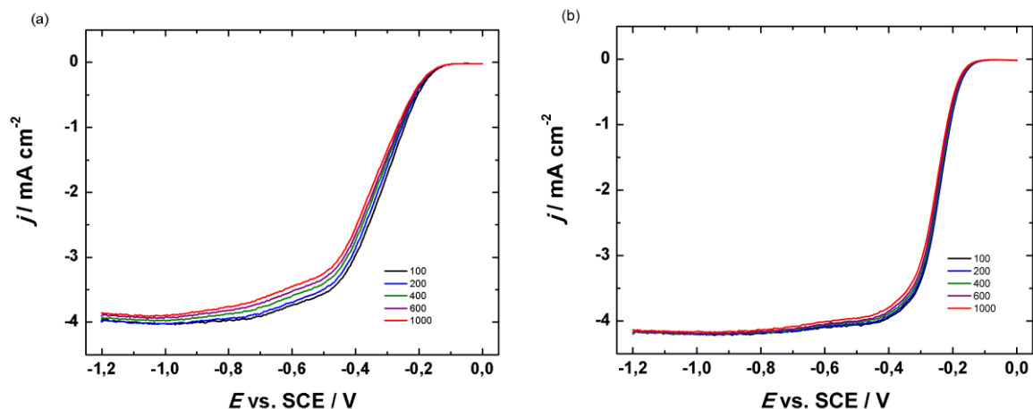
Joonis 9. (a) FeNCNS materjaliga modifitseeritud klaassüsinikelektroodi polarisatsioonikõverad hapnikuga küllastatud 0,1 M KOH lahuses pärast 100, 200, 400, 600 ja 1000 tsüklit laotuskiirusega 100 \text{mV s}^{-1} . (b) CoNCNS materjaliga modifitseeritud klaassüsinikelektroodi polarisatsioonikõverad. \nu = 10 \text{ mV s}^{-1} , \omega = 1900 \text{ p min}^{-1} .
