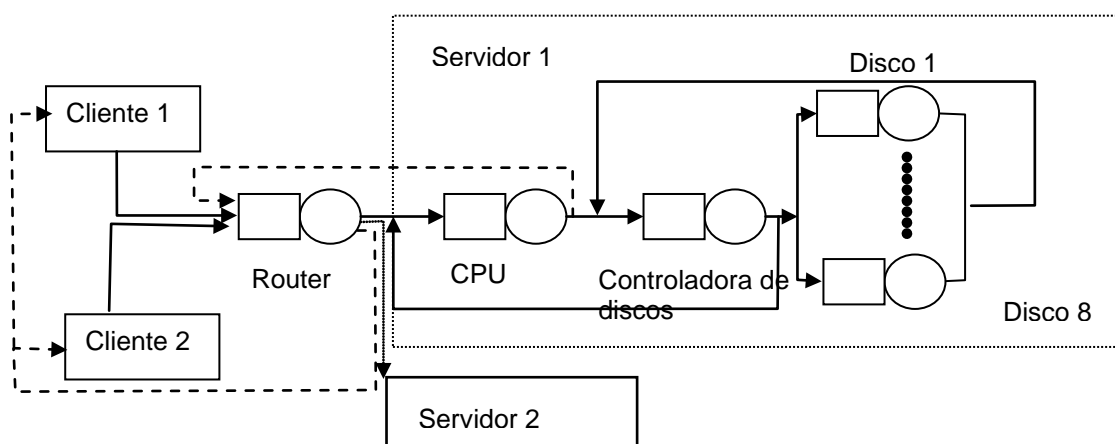
Figura 2: Modelo Cliente/Servidor con descripción detallada de estructura del servidor
