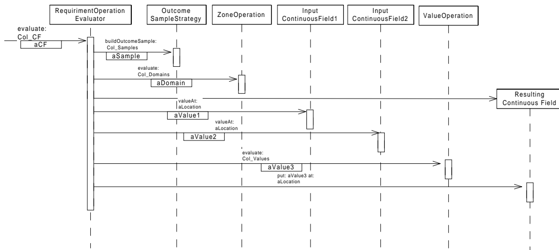
Figura 9 Diagrama de Interacción: una etapa de evaluación
