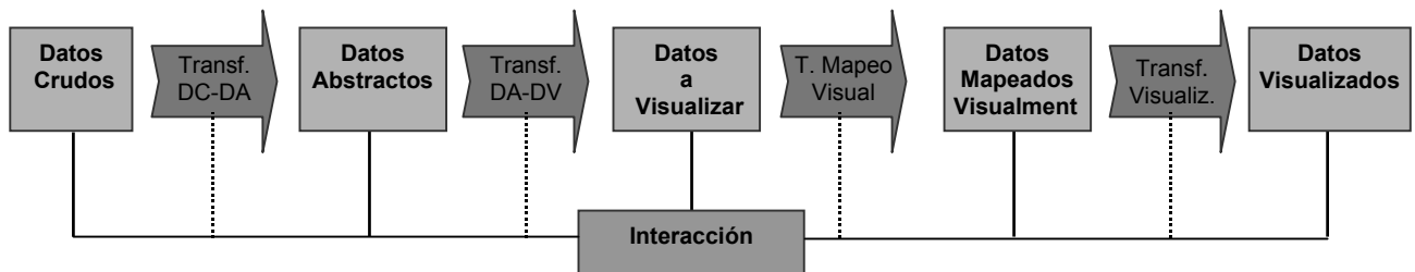
Fig. 2: Modelo Unificado de Visualización
