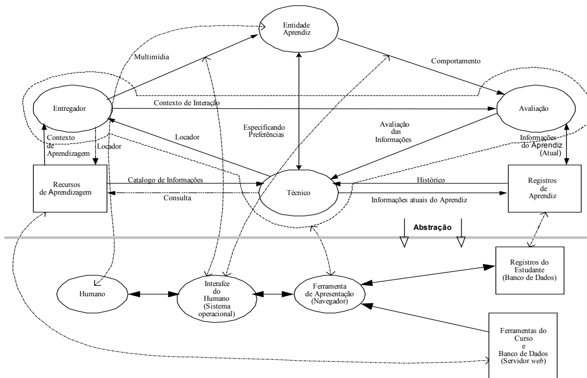
Figura 8 – Sistema Hipotético Mapeado para o Modelo IEEE/LTSA.
