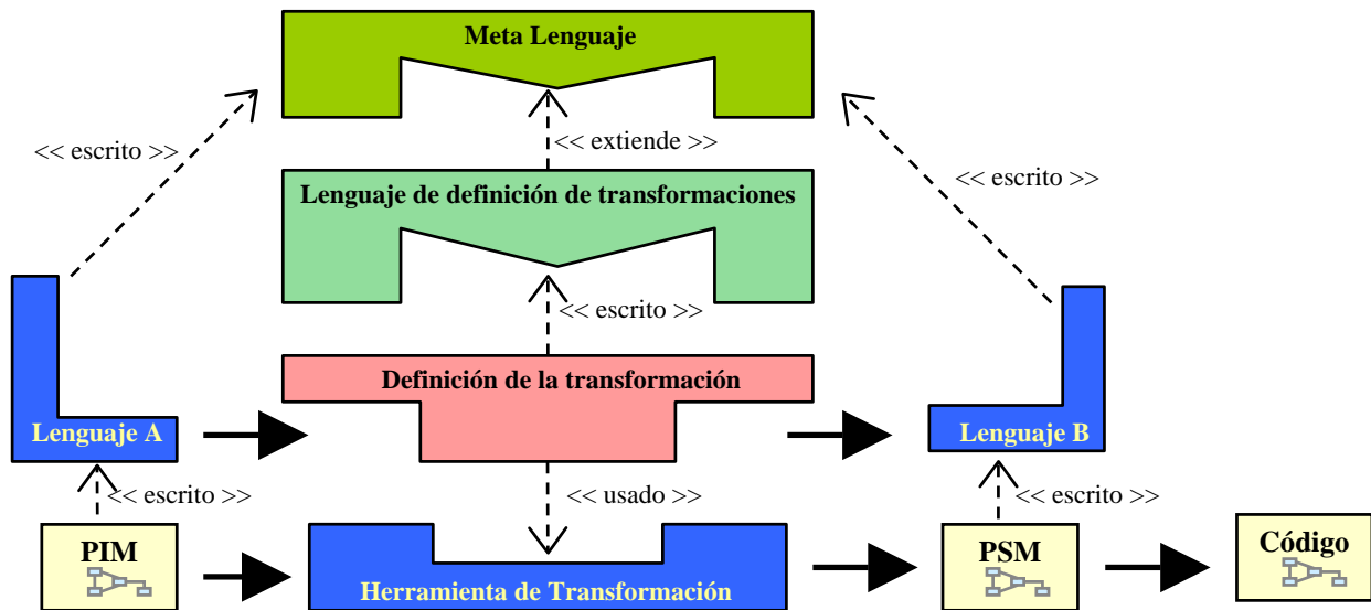
Figura 2: Integración de los componentes del framework
