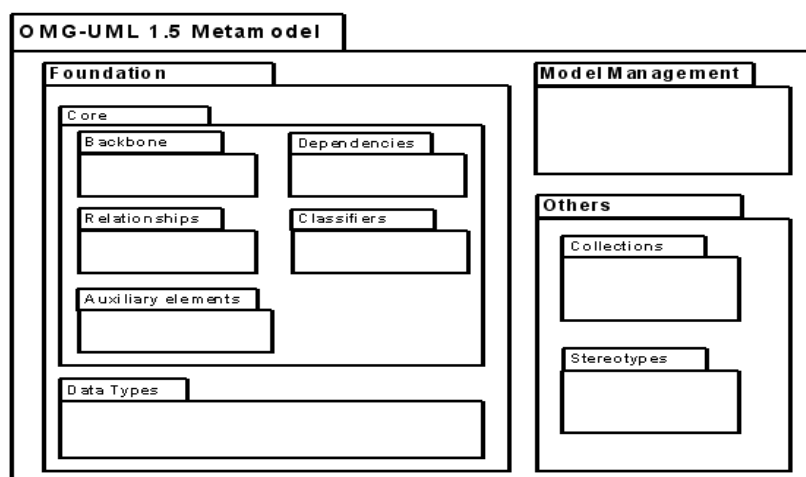
Figura 8: Paquetes del Metamodelo
