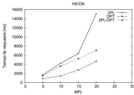
Figura 16: Tiempo de Respuesta para la carga HICON
