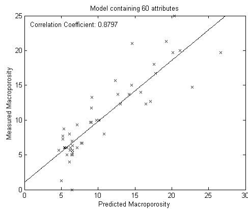
Fig. 3. Correlação entre os valores preditos com o modelo de 60 atributos e os valores reais.
