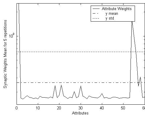
Fig. 1. Escores para cada um dos 60 atributos de entrada.
