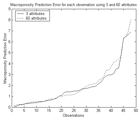
Fig. 2. Erros de predição de macroporosidade com 3 e 60 atributos de entrada.
