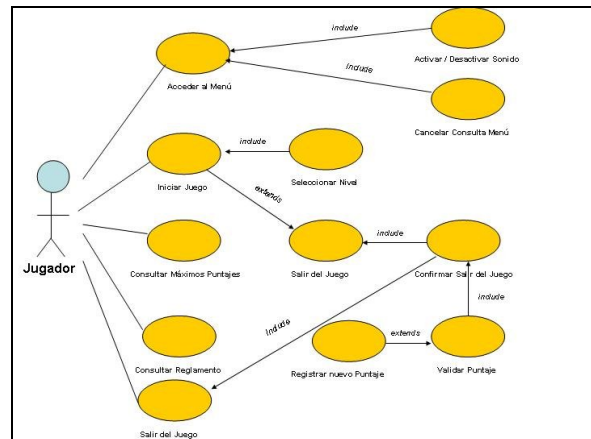
Fig. 1: Diagrama de casos de uso del juego simple.
