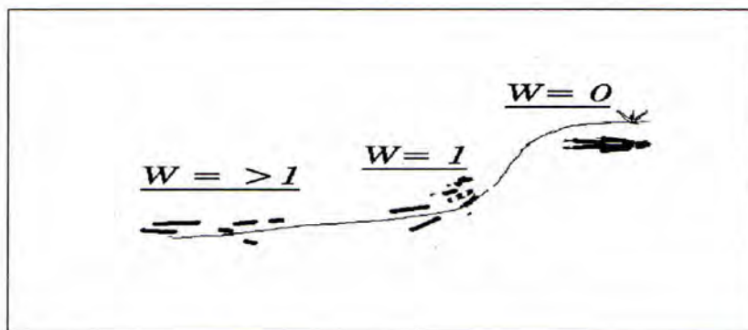
Figura 2. Esquema sobre las expectativas de avance en el grado de meteorización ( W ) en relación a su ubicación en las diferentes cotas
