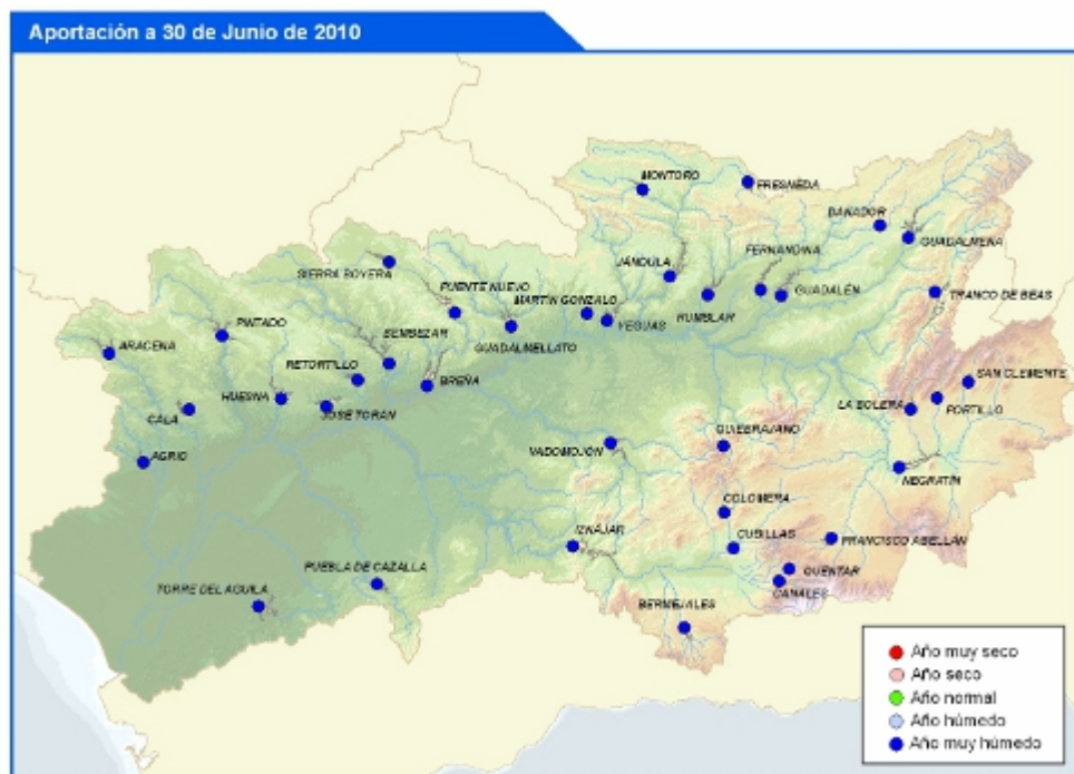
Figura 8. Imagen de estado hidrológico a finales de junio del año hidrológico 2009/10.
