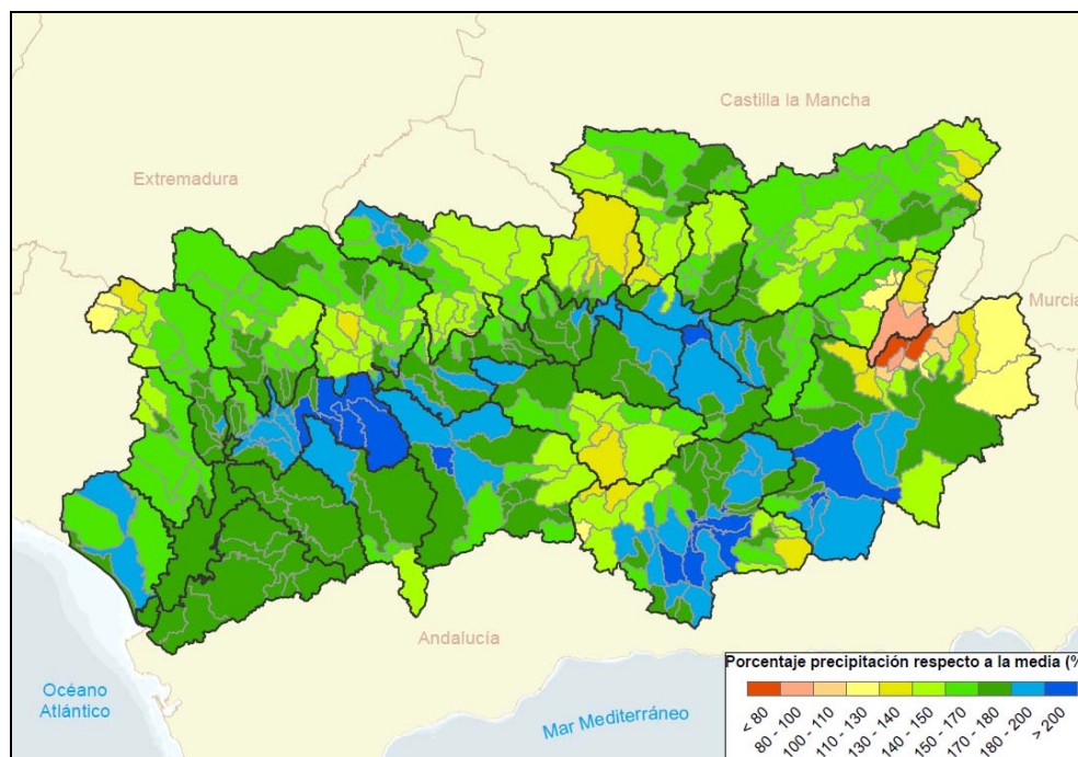
Figura 10. Precipitación acumulada a 30 de junio de 2010 con respecto a la media
