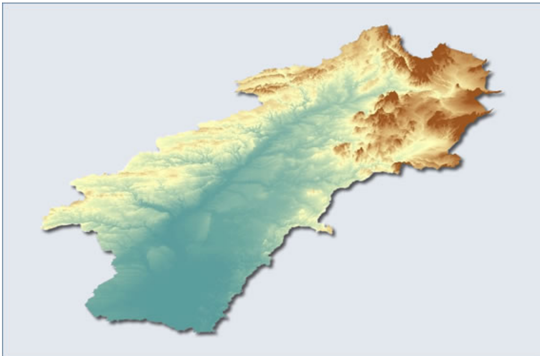
Figura 5. Modelo de elevaciones de la cuenca del Guadalquivir
