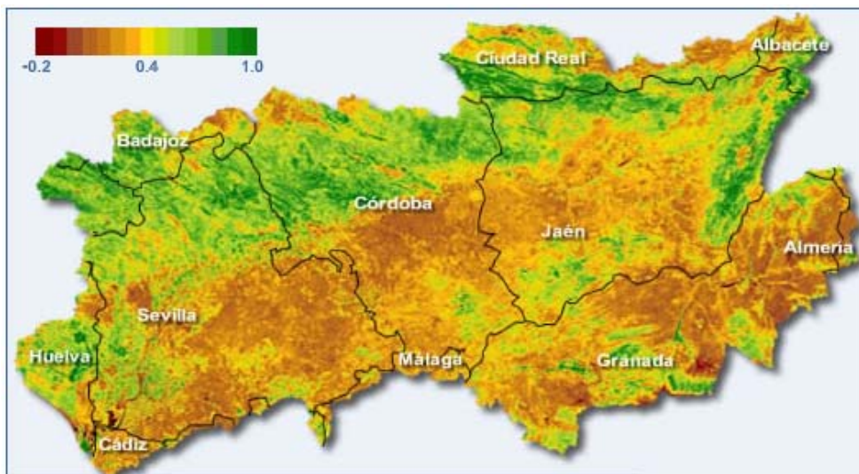
Figura 7. Imagen NDVI de la cuenca
