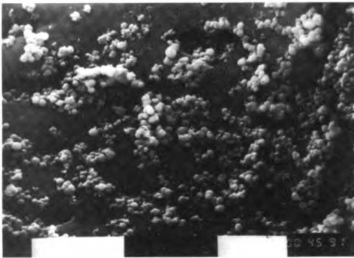
Figura 2. Microfotografía con MEB. Populus deltoides cv A-568-1. Depósitos hemisféricos del preservante. Escala: 10 \mu m
