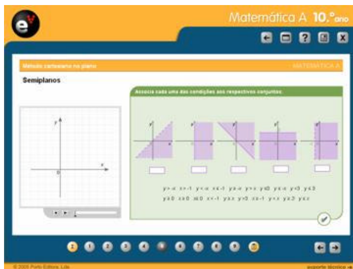
Figura 3.7 – Semi-planos
