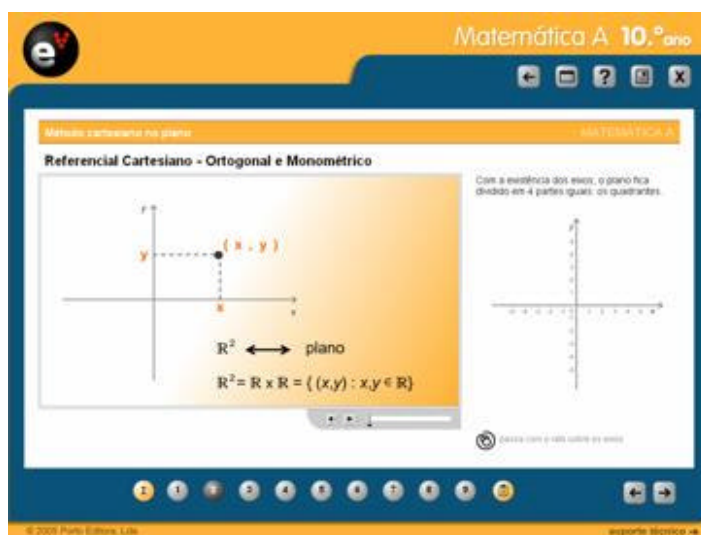
Figura 3.2 – Referencial cartesiano
