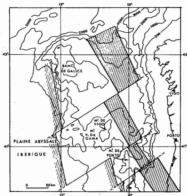
Fig. 2 — Répartition schématique des bassins du Mésozoïque inférieur sur la marge au Nord-Ouest de la Péninsule Ibérique (d'après MAUFFRET et al., 1978)
