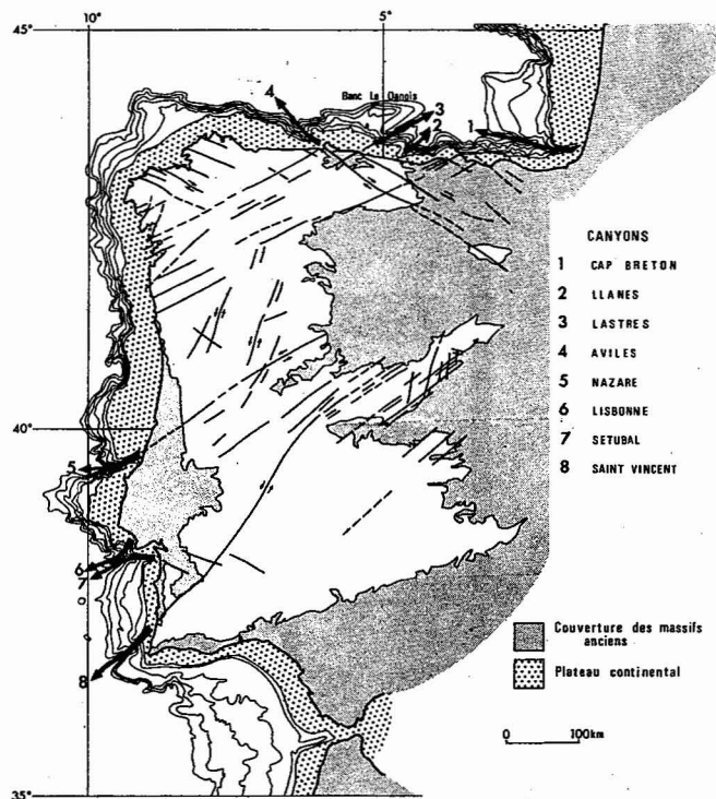
Fig. 1 — La situation des grands canyons sous-marins de la Péninsule Ibérique et leurs relations avec les décrochements «tardihercyniens» (d'après BOILLOT et al., 1974; et d'après PARGA, 1969, modifié)
