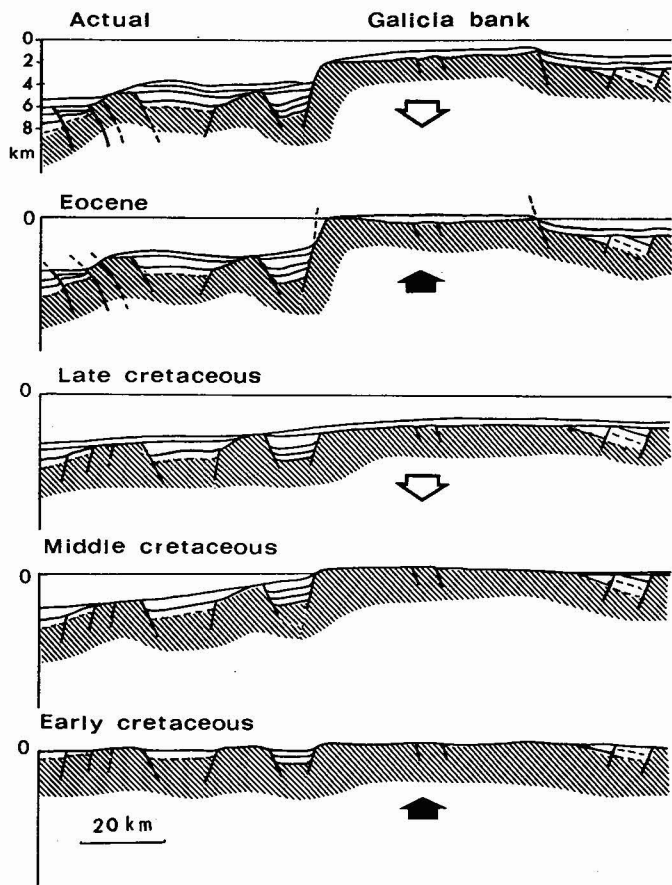
Fig. 3 — Évolution structurale de la montagne de Galice, au Nord-Ouest de la Péninsule Ibérique (la coupe est orientée E-W, et située approximativement sur le parallèle 42° 40' N (d'après BOILLOT et al., 1979a, simplifié)
