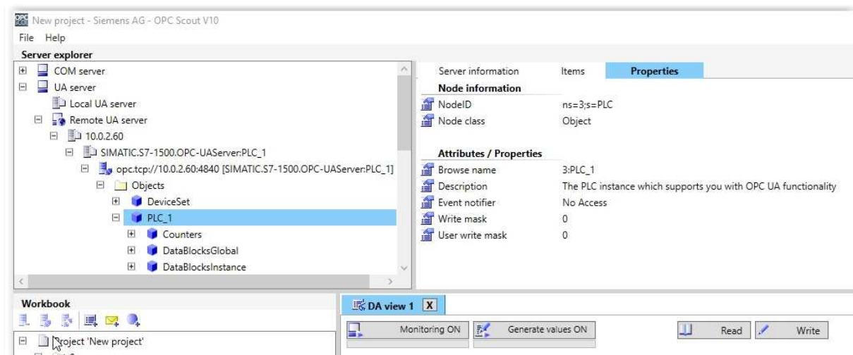
Fig. 20 : Connexion au serveur OPC UA de l'API (PLC_1)
