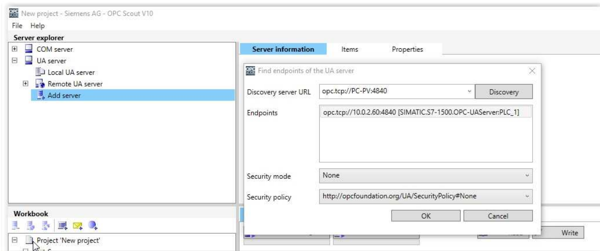
Fig. 17 : Connexion au serveur OPC UA de l’API ( opc.tcp://10.0.2.60 :4840 )
