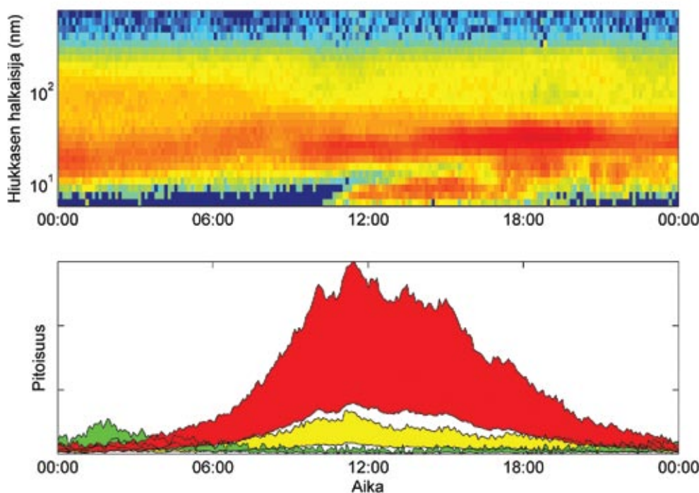
Kuva 5. Hiukkasten kokojakauma (yläpaneeli) ja eräiden tiivistymiskykyisten höyryjen pitoisuuden vaihtelu Aboalla tammikuuisena päivänä 2015. Hiukkasmuodostustapahtumanalku havaitaan hieman ennen keskipäivää. Hiukkasmuodostus erottuu yläpaneelin kuvassa punaisella värillä hiukkasten halkaisijan kasvaessa hitaasti. Alapaneelistä nähdään, että tiivistymiskykyisten höyryjen pitoisuus kasvaa samanaikaisesti.
