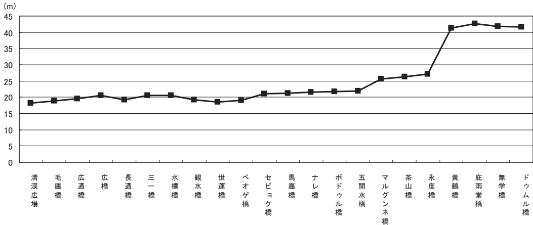
図5 清溪川における護岸幅の計測結果
