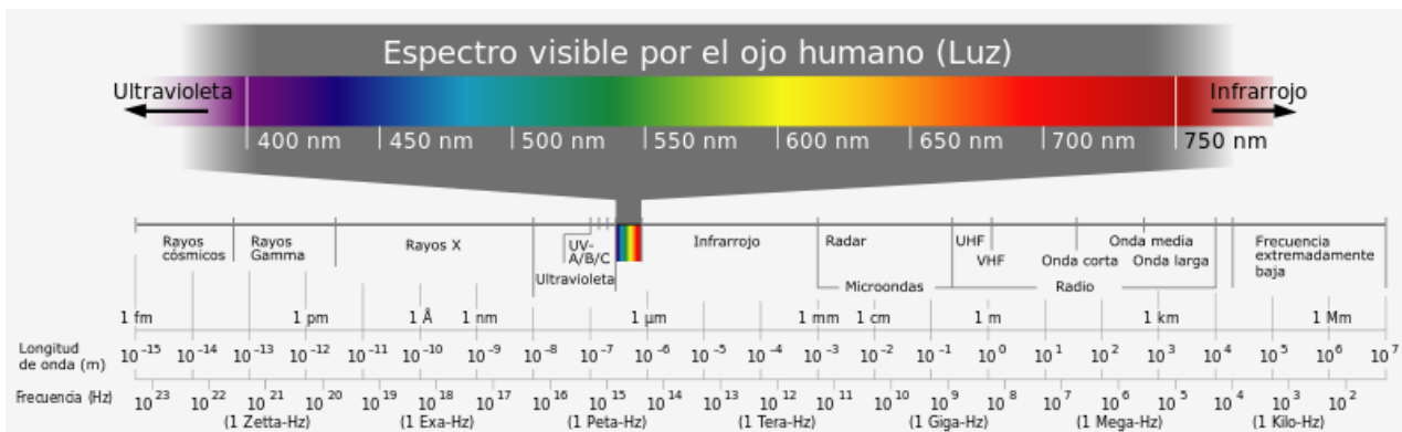
Figura 1.5. Esquema del espectro electromagnético.
