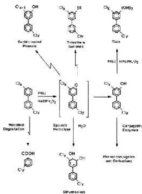
Slika 8.: Raspad PCB-a pod utjecajem mikroorganizama
