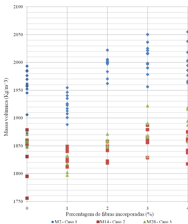
Figura 4: Massas volúmicas às idades de 2 dias, de 14 dias e de 28 dias, com fibras de 2 cm de comprimento
