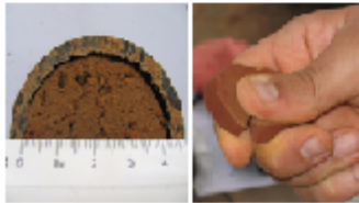
Figura 3 – ‘Teste da pastilha’ - procedimentos e critério de avaliação de adequabilidade do solo habitualmente utilizados nas construções.
