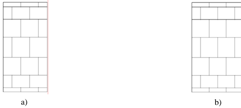
Figura 7. Planta de um arco com diferentes opções de assentamento: a) um meio bloco por fiada; b) dois meios blocos em fiadas intercaladas.
