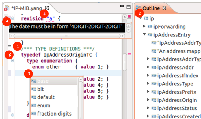
Figure 4: Yang plugin editor
