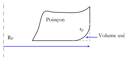
FIG. 2 - Géométrie de l'arête coupante du poinçon.
