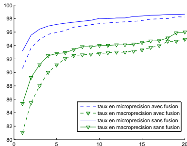
FIG. 7 – Courbes CMC ; les courbes en lignes pleines représentent les taux obtenus dans l'espace \Omega_{sf} et les courbes en pointillés ceux dans l'espace \Omega_{af} .
