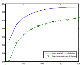
FIG. 8 – Evolution des taux de reconnaissance sur \Omega_{sf}^{ACPX} en fonction de la dimension X .
