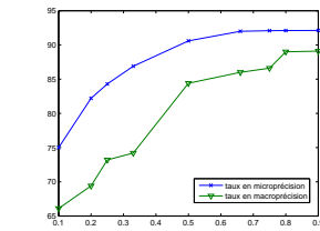
FIG. 9 – Evolution des taux de reconnaissance (dans \Omega_{af} ) en fonction de la proportion d'échantillons.
