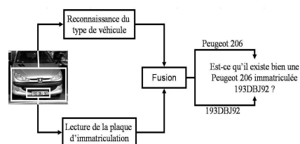
FIG. 1 – Système d'identification de véhicule fusionnant la reconnaissance de son type et la lecture de sa plaque d'immatriculation.
