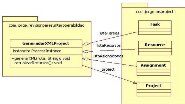
Figura 28. Diagrama de clases paquete com.jorge.revisionpares.interoperabilidad.
