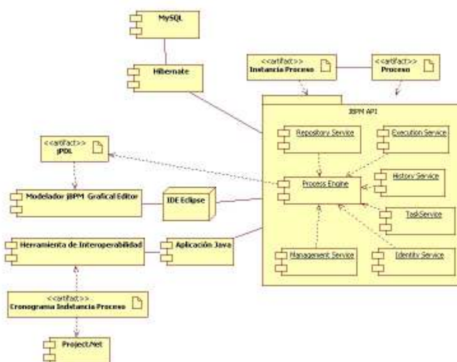
Figura 17. Vista de despliegue solución en JBPM.
