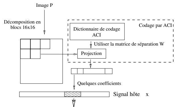
FIG. 4 – Codage d'une image P par ACI
