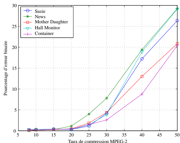
FIG. 6 – Robustesse de la méthode utilisant l'ACI face à une compression MPEG-2
