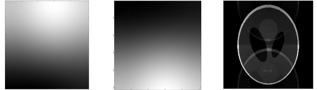
FIG. 4 : à gauche, les sensibilités estimées par la méthode ICASENSE puis lissées et interpolées, à partir des acquisitions de la figure 3. A droite, l'image reconstruite à partir de ces données et des images figure 3, en inversant l'équation (1).
