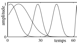
FIG. 5: Fenêtres gaussiennes obtenues pour 5 attributs qui sont des moments d'ordre 1
