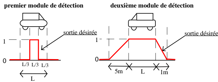
figure 2 : Sorties désirées des modules de détection. L désigne la longueur du véhicule.
