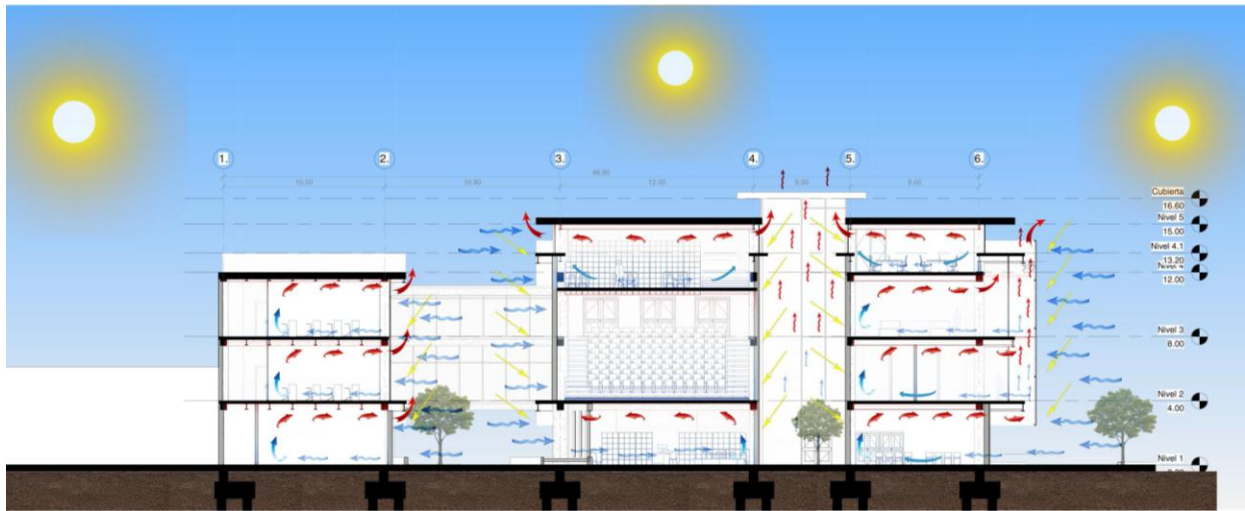
Figura 18- Ventilación Cruzada
