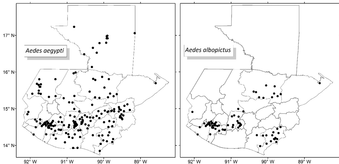
Figura 1. Presencia de vectores de arbovirus en Guatemala. Izquierda: Localización geográfica de Aedes aegypti (puntos negros) en 21 de los 22 departamentos del país. Tonicapán fue el único departamento en donde no se reporta esta especie de vector a la fecha. Derecha: Reportes de Aedes albopictus (puntos negros). Reportes para esta especie no fueron encontrados en 11 departamentos de Guatemala.
