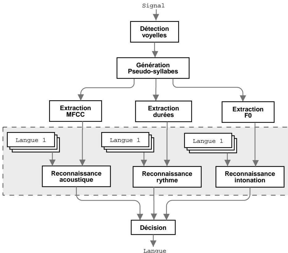
Figure 3. Schéma synoptique du système global d'identification des langues.
