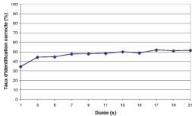
Figure 6. Taux d'identification correcte pour le système «skewness/kurtosis».
