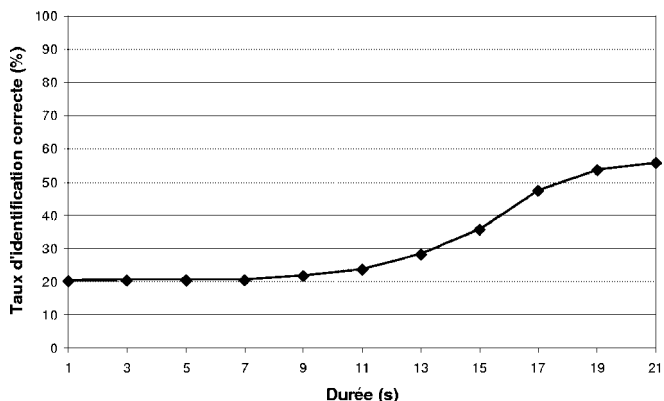
Figure 7. Taux d'identification correcte pour le système « place de l'accent ».
