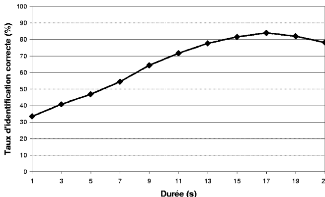
Figure 8. Fusion du système « skewness/kurtosis » et du système « place de l'accent ».
