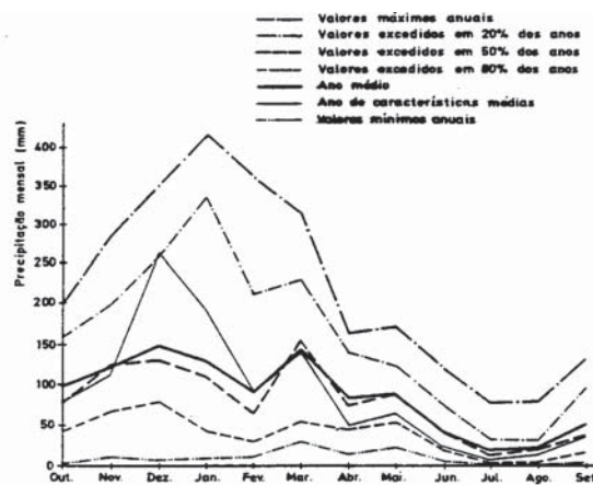
Figura 4.24 Distribuição mensal das precipitações na bacia do Mondego em Ponte de Tábua (Qintela, 1992).
